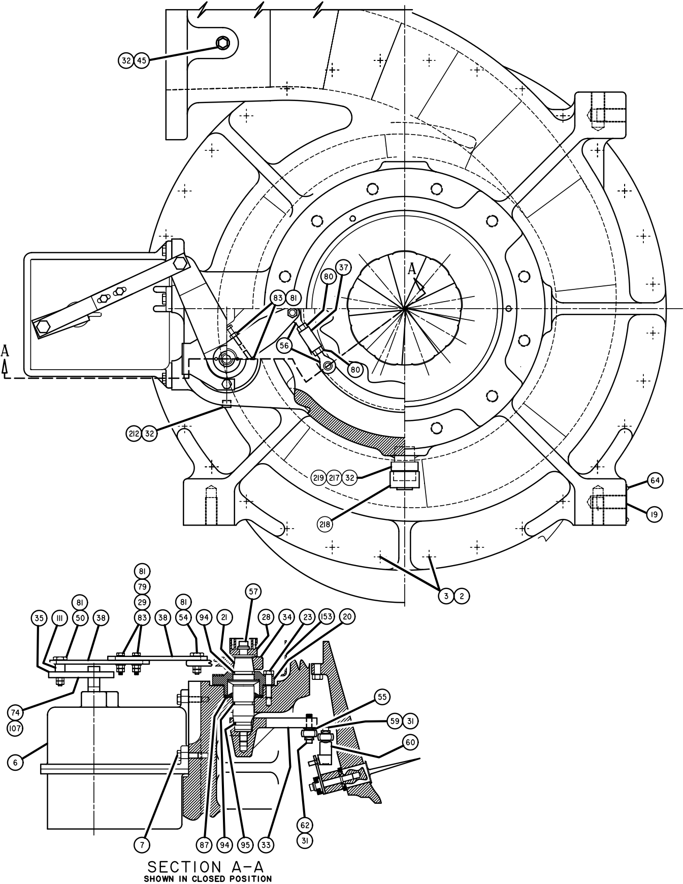
FIG. 3 – HA COMPRESSOR (41)
