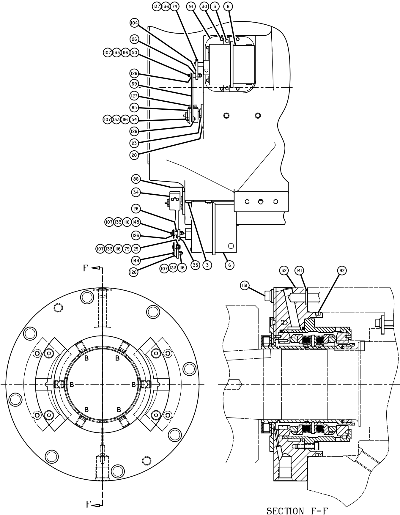
FIG. 54 – HA COMPRESSOR (119)
