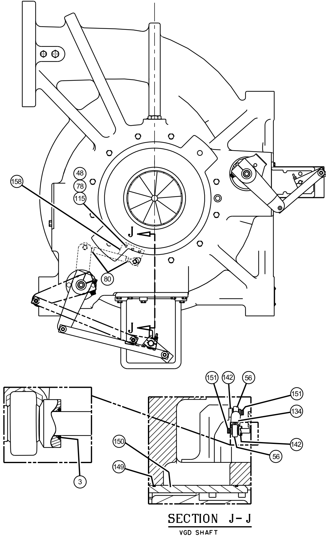
FIG. 47 – HA COMPRESSOR (81, 90, 104)
