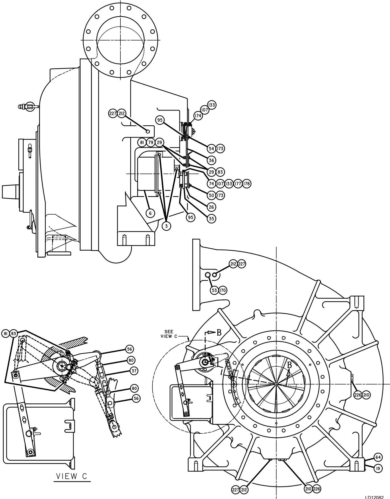
FIG. 45 – HA COMPRESSOR (81, 90, 104)
