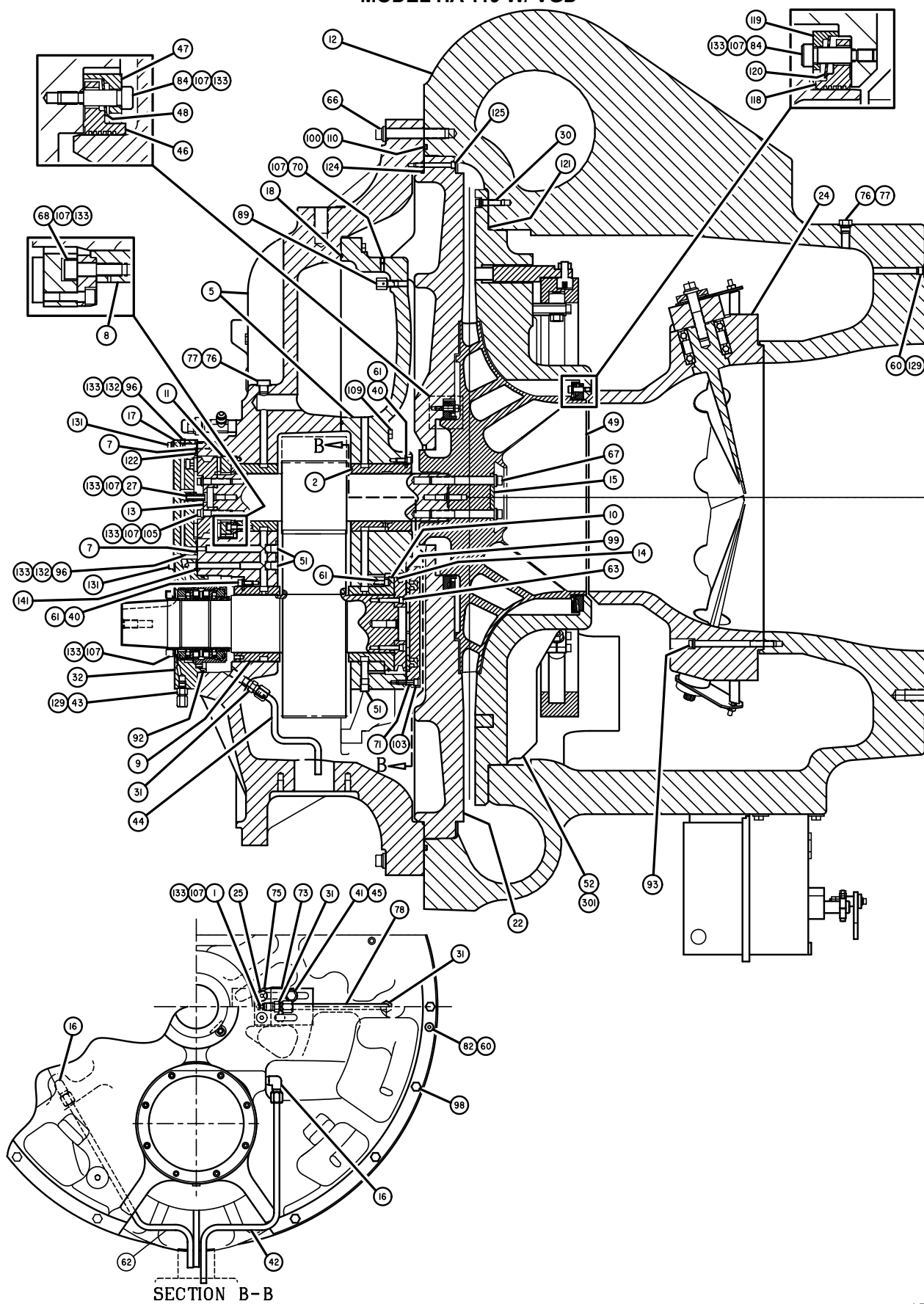
FIG. 51 – HA COMPRESSOR (119)
