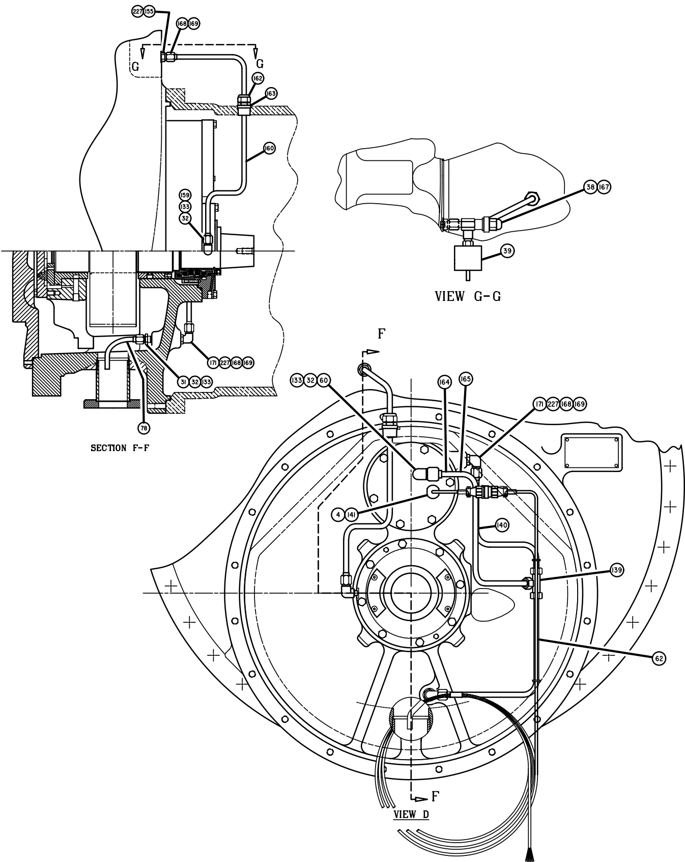
FIG. 46 – HA COMPRESSOR (81, 90, 104)
