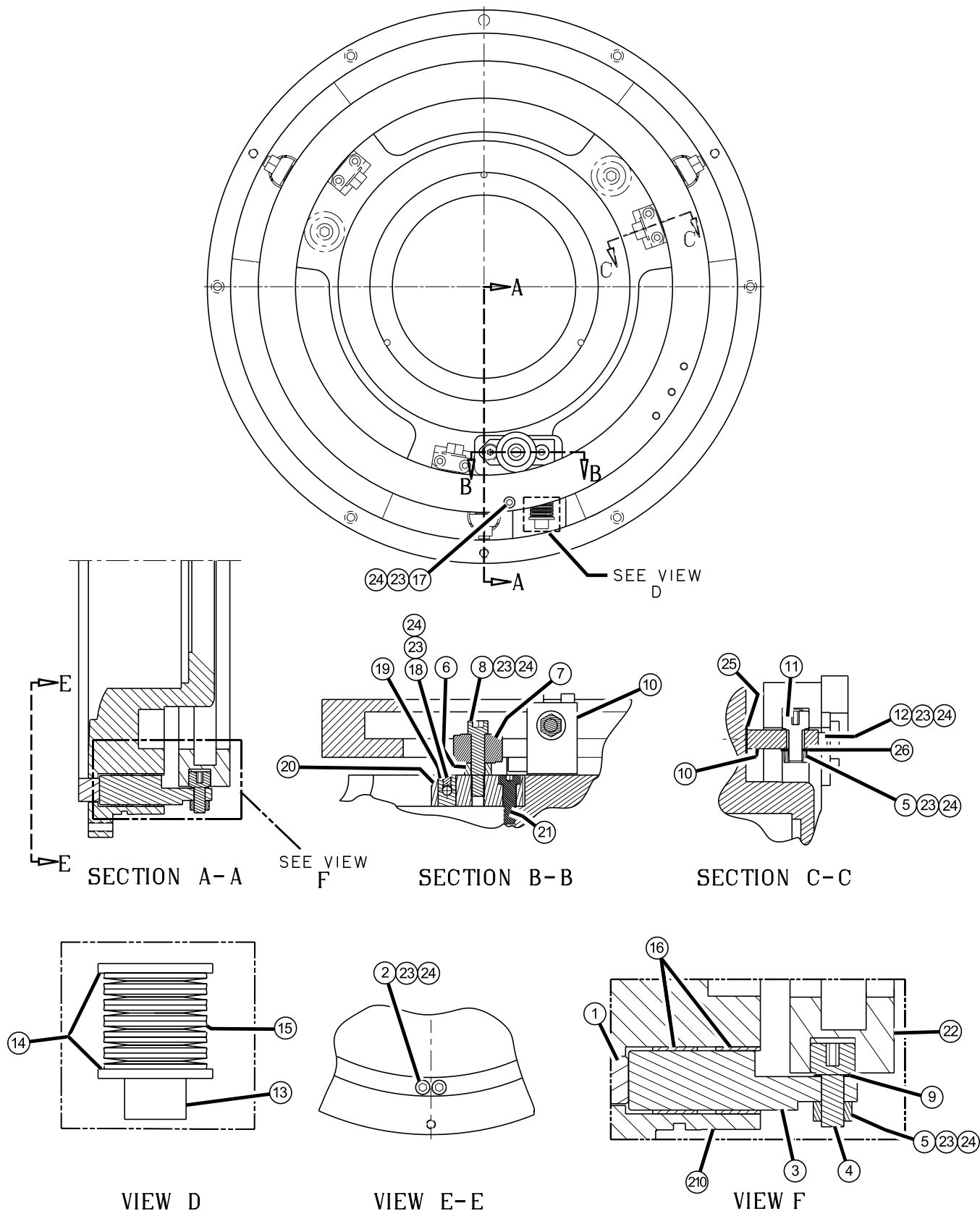
FIG. 26 – VGD DEVICE (HE 70)
