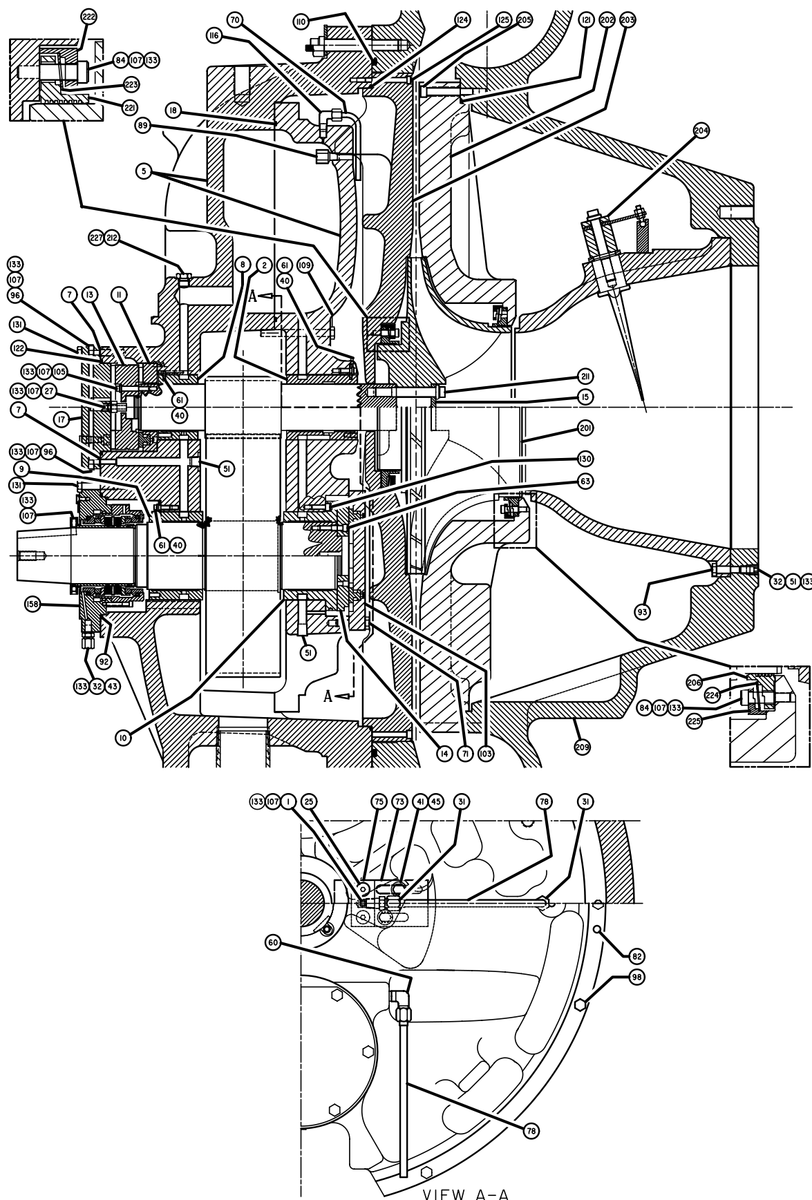
FIG. 43 – HA COMPRESSOR (81, 90, 104)
