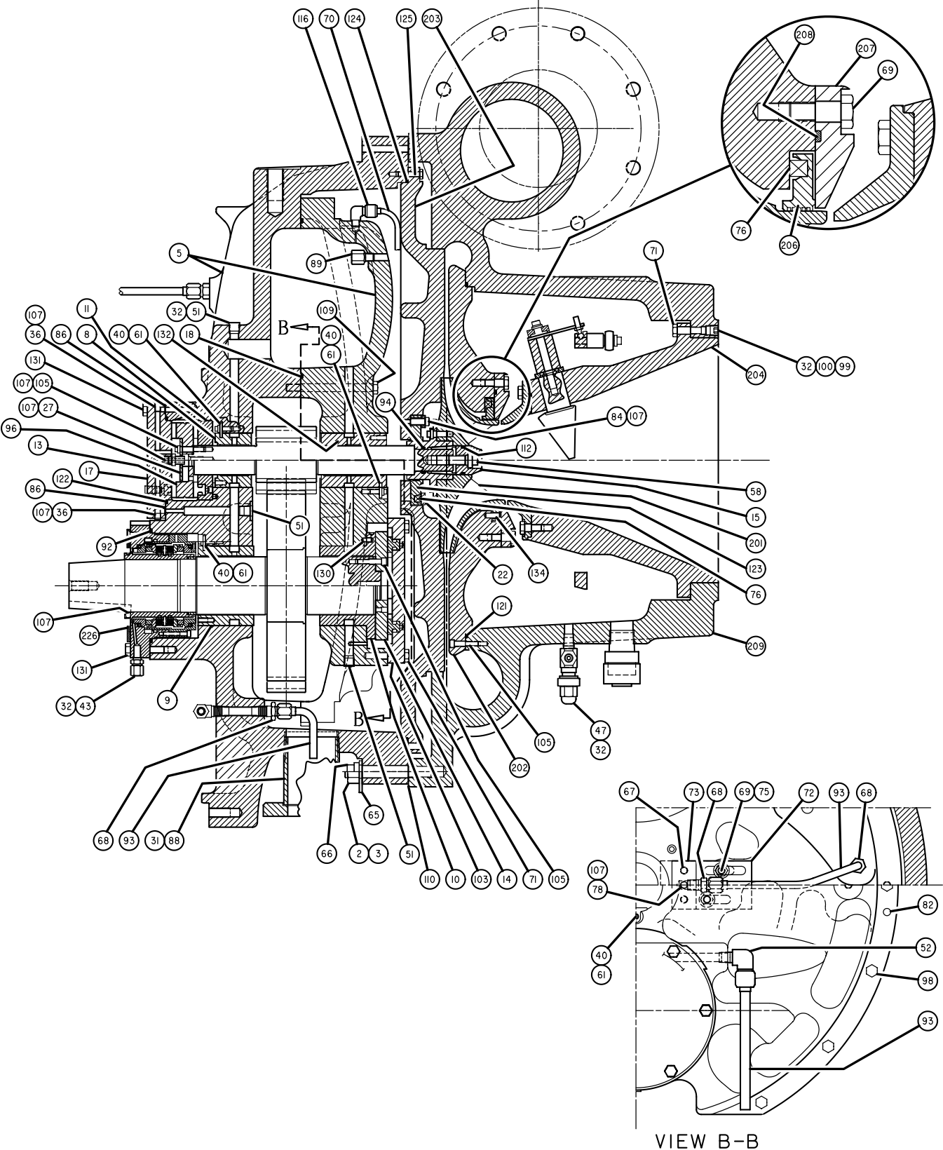
FIG. 1 – HA COMPRESSOR (41)
