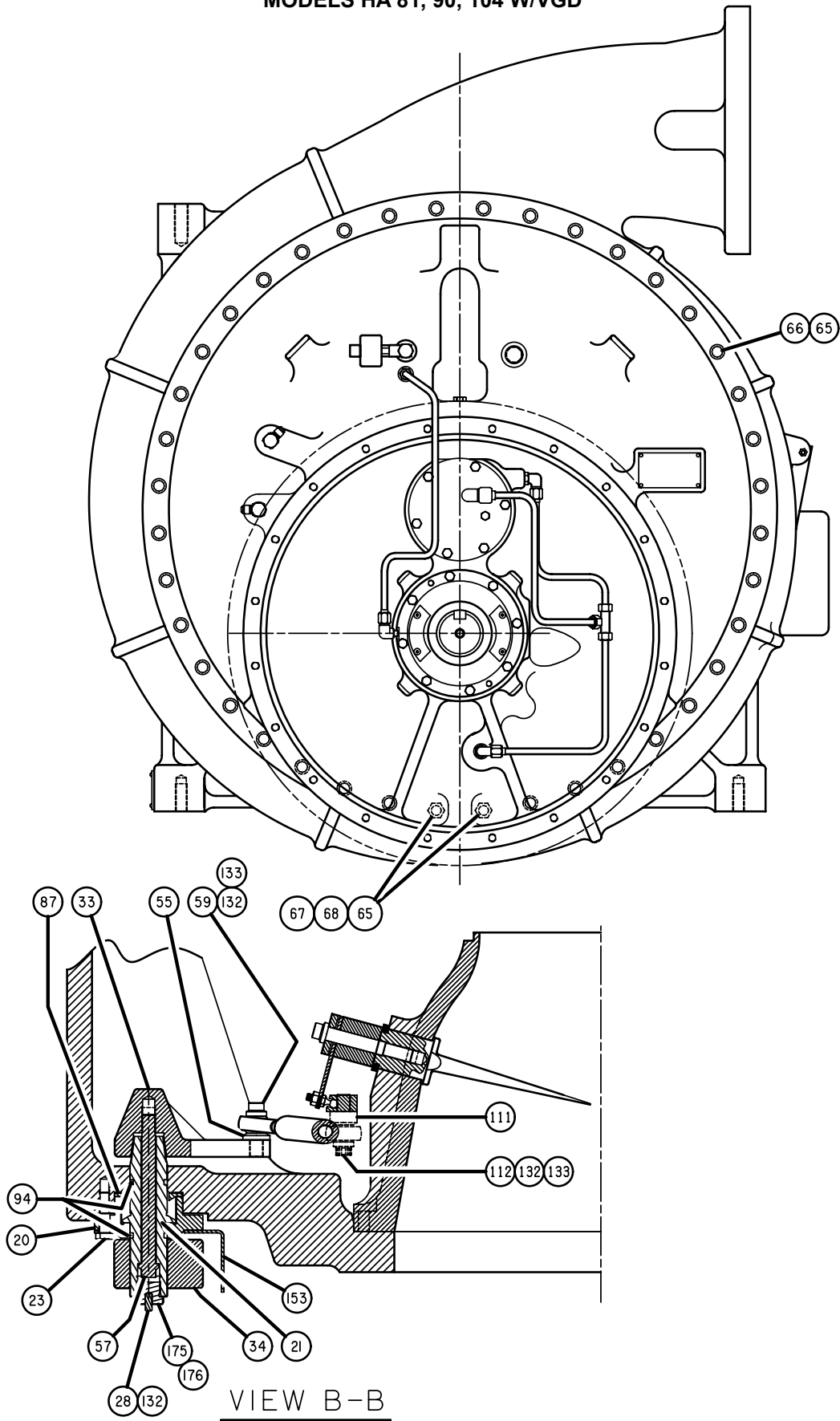
FIG. 44 – HA COMPRESSOR (81, 90, 104)
