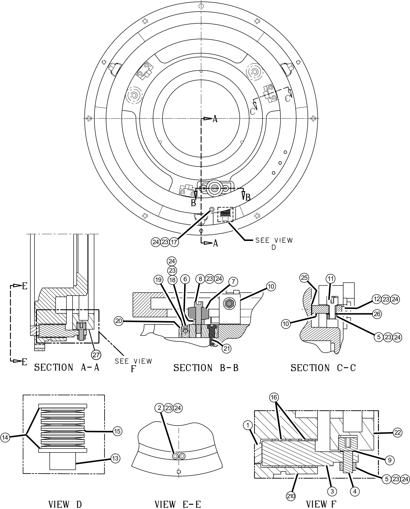
FIG. 36 – VGD DEVICE (HG 65, 73)
