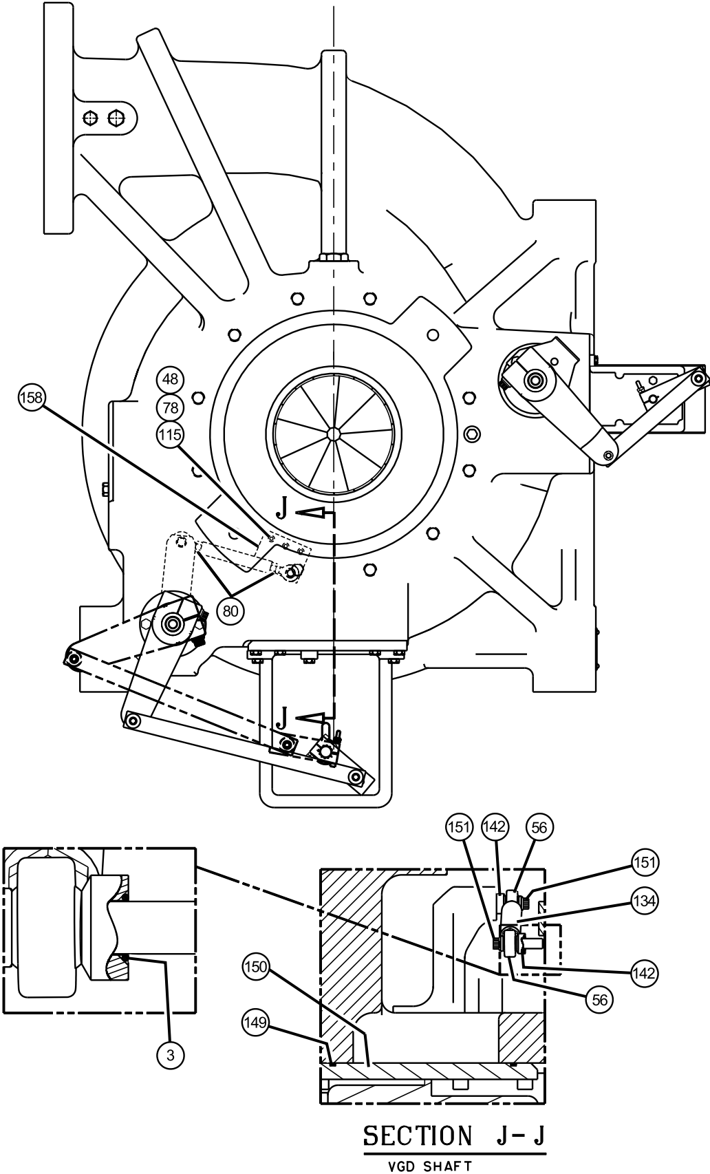
FIG. 24 – VGD DEVICE (HE 70)
