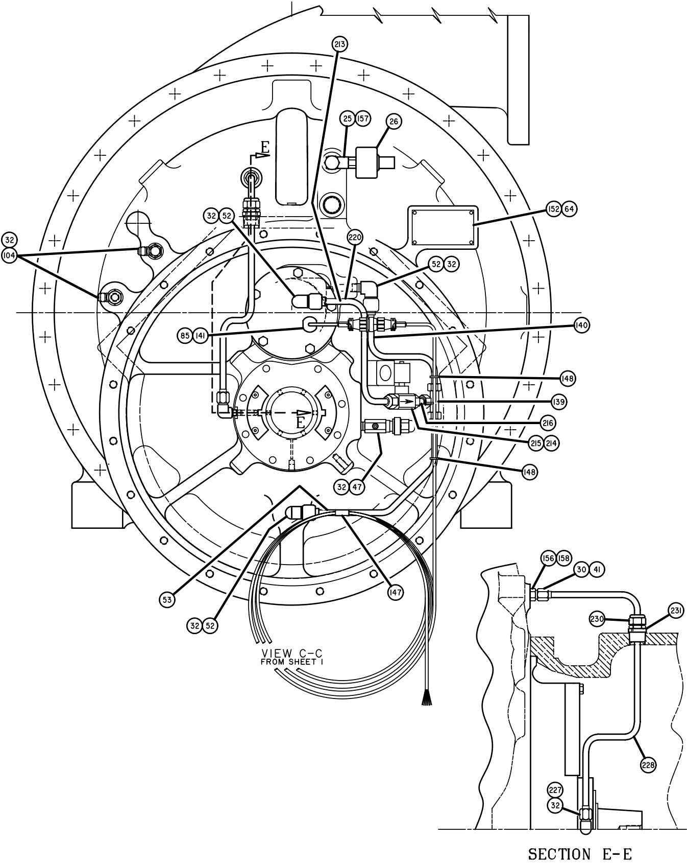
FIG. 2 – HA COMPRESSOR (41)
