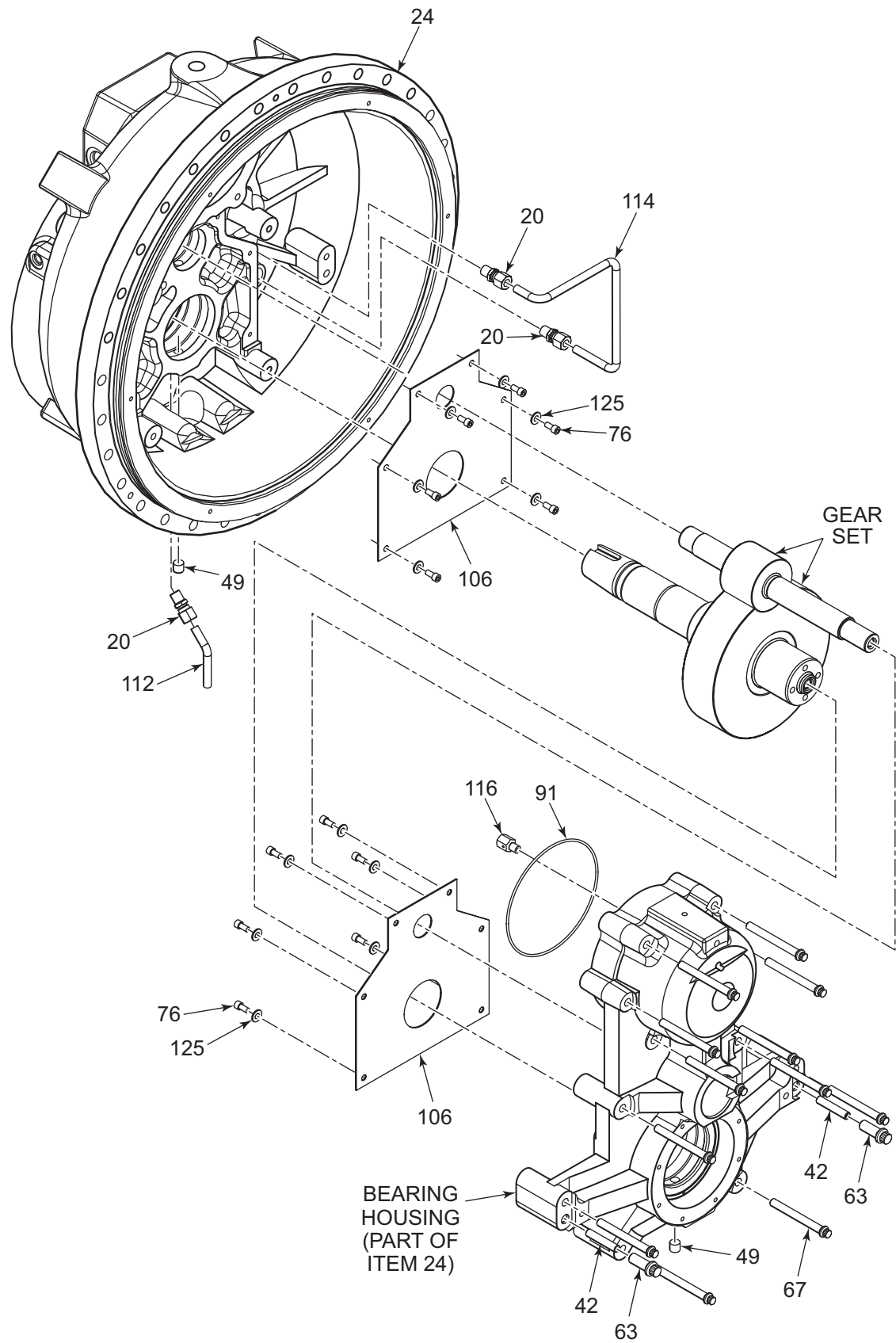
FIG. 11 - HF 41 COMPRESSOR
