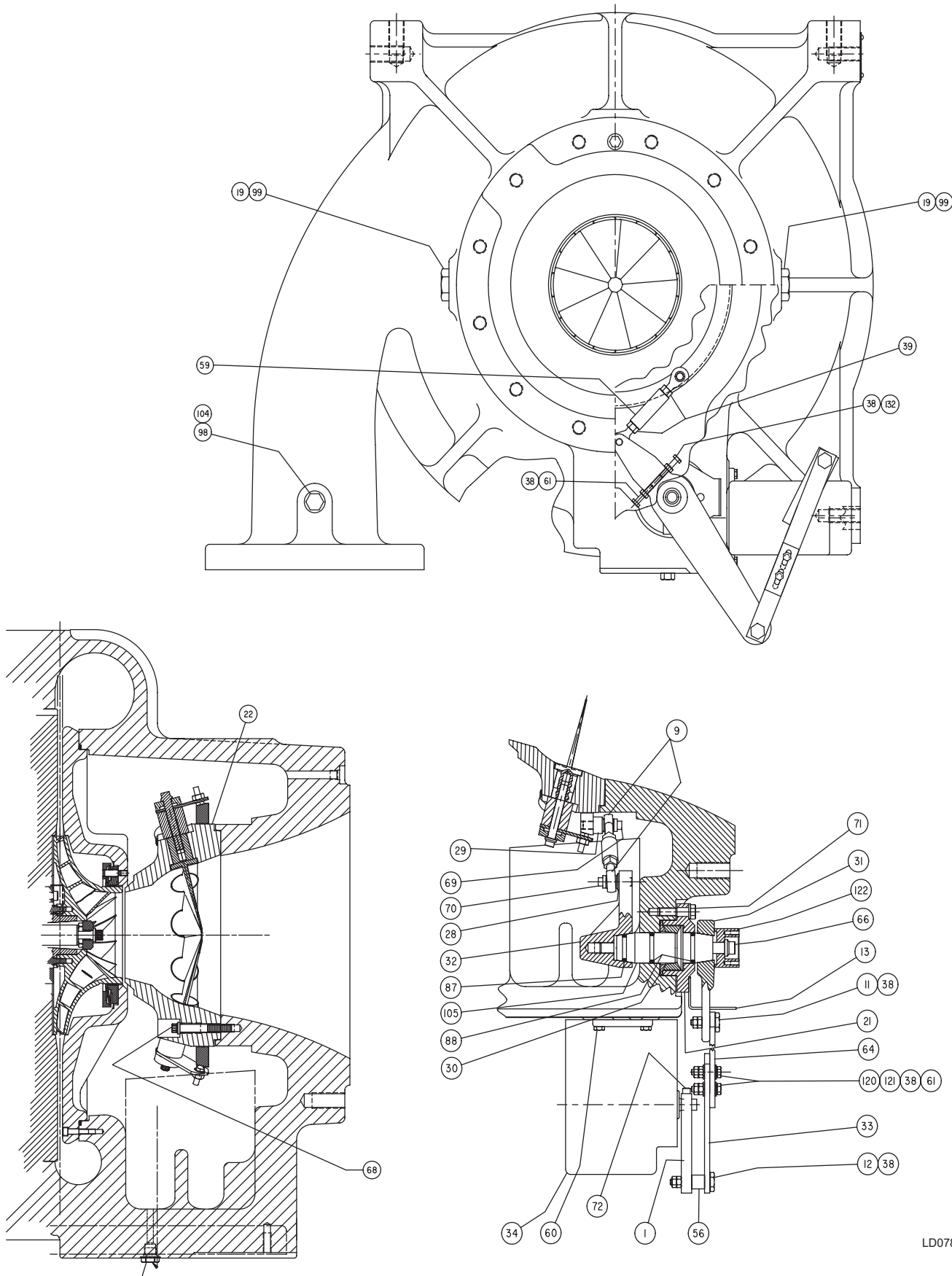
FIG. 14 - HF 41 COMPRESSOR
