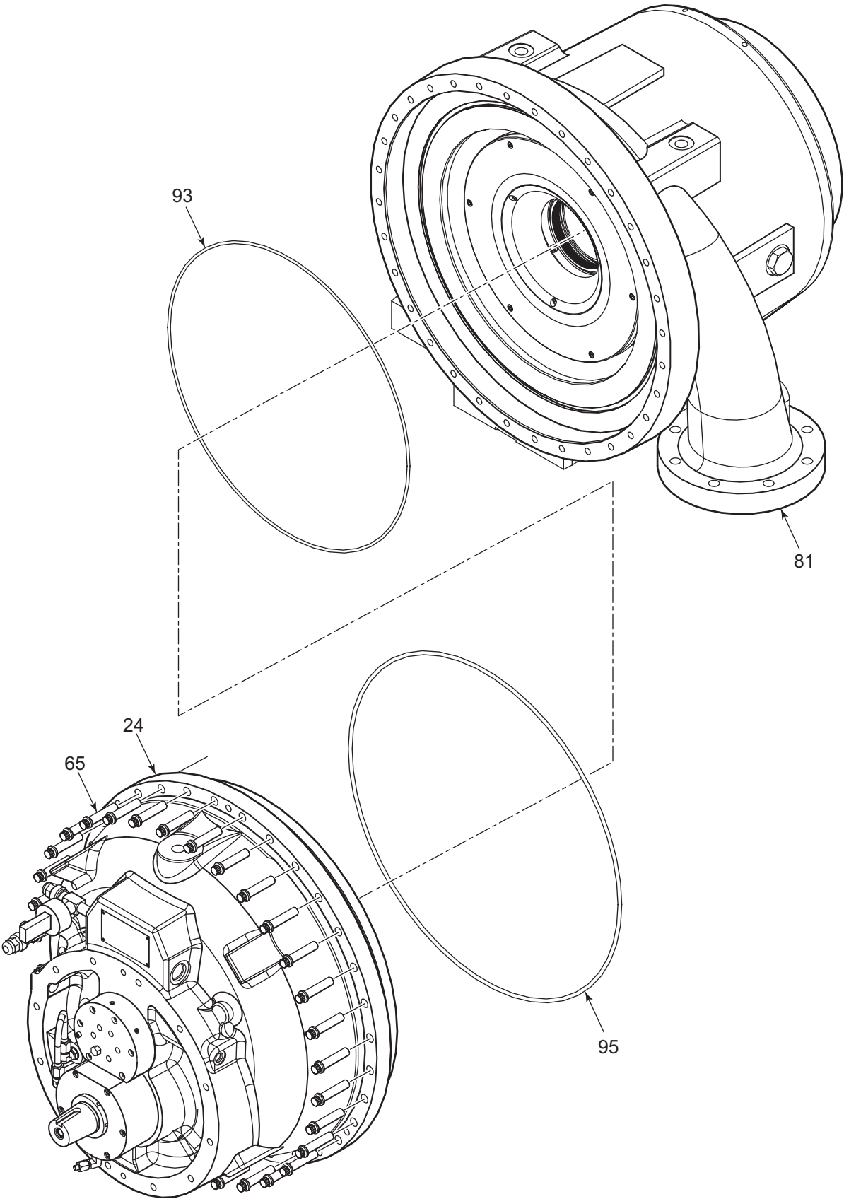
FIG. 12 - HF 41 COMPRESSOR
