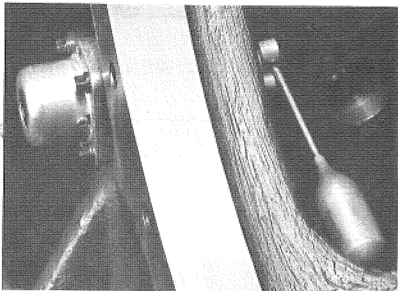
FIG. 14— FLOAT SWITCH
