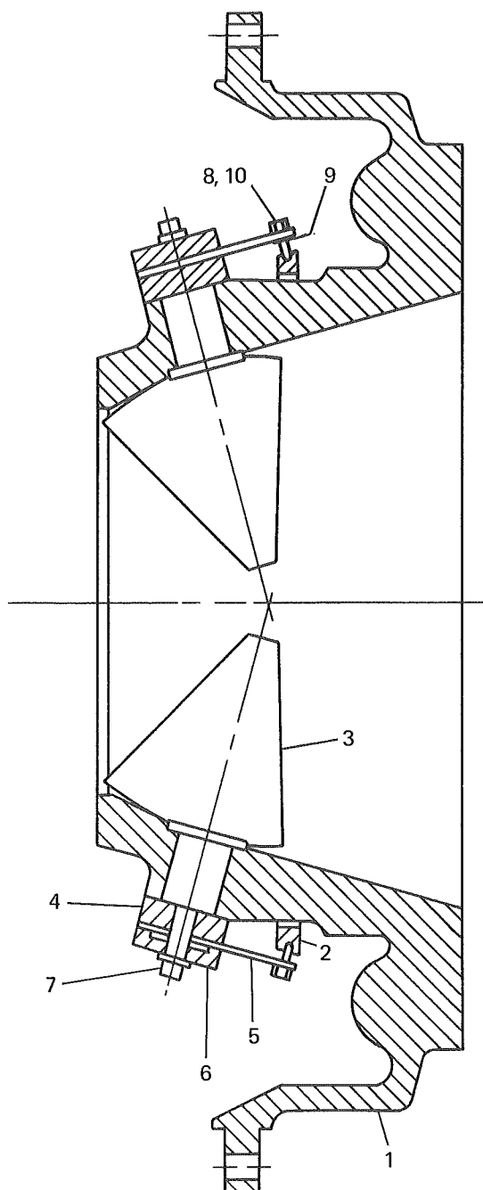
FIG. 7— PRV ASSEMBLY
