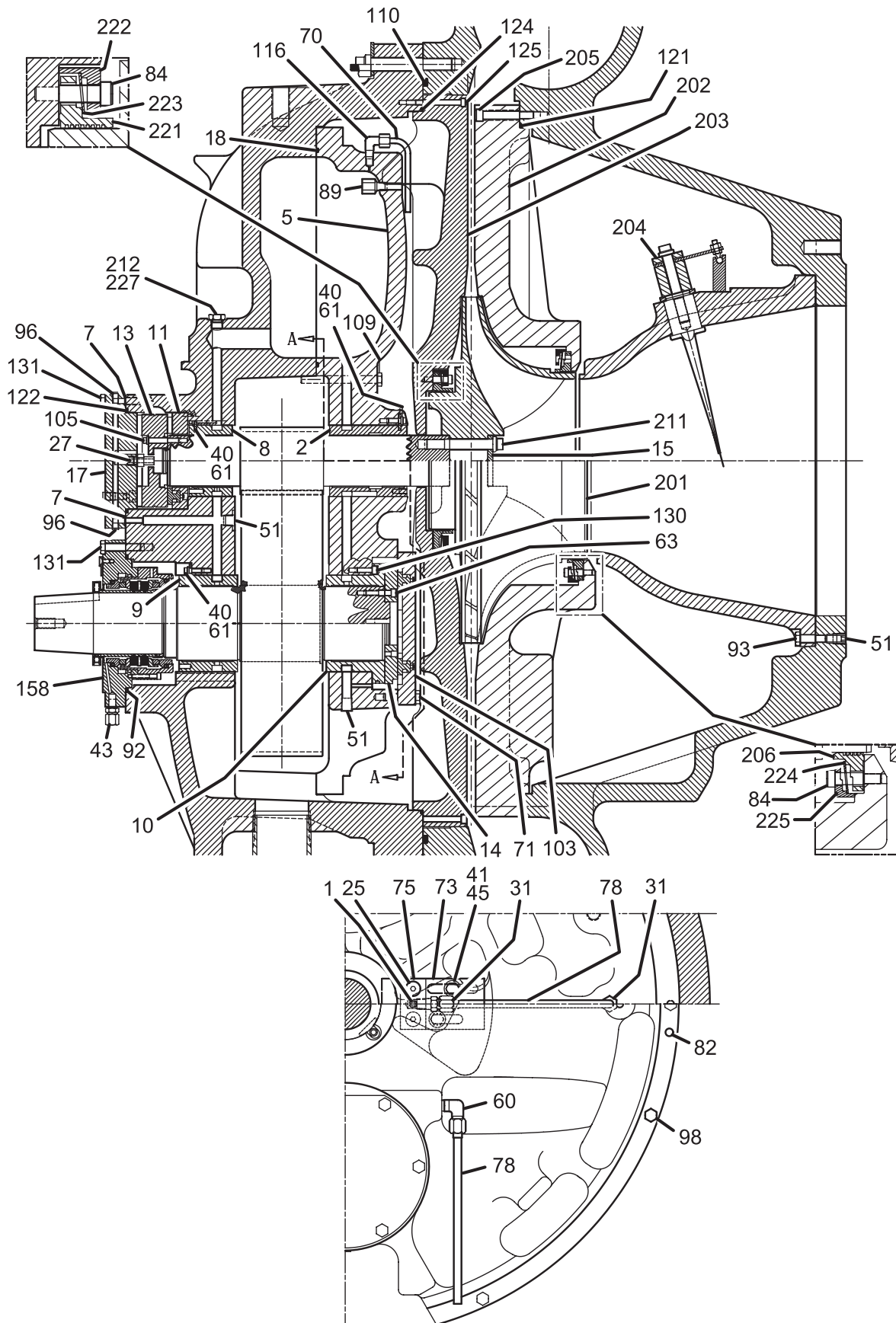
SECTION A-A
