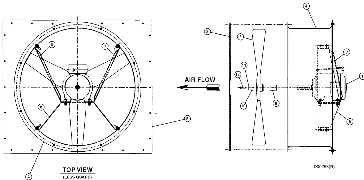
FIG. 6 – FAN – Typical
