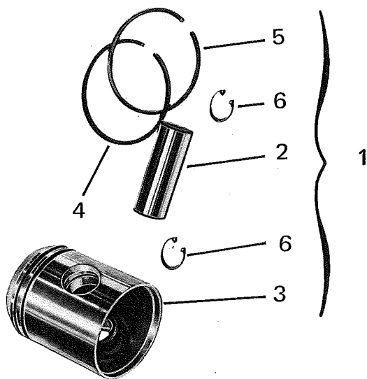
FIG. 3- PISTON
