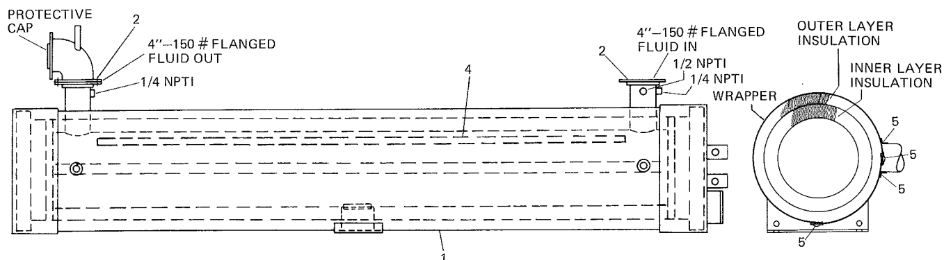
FIG. 6—COOLER
