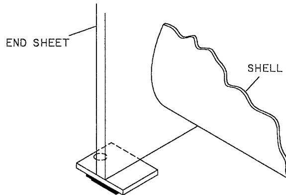
NEOPRENE PADS
