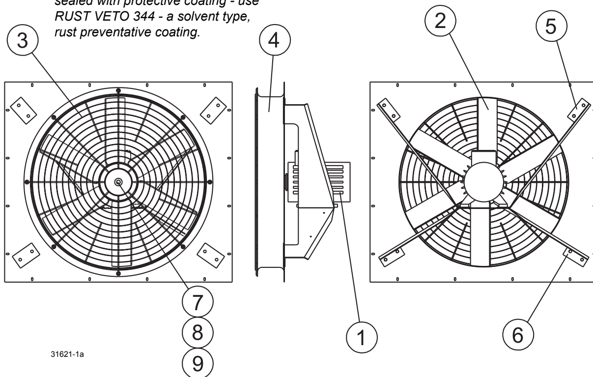
FIG. 3a – FAN COMPONENTS
