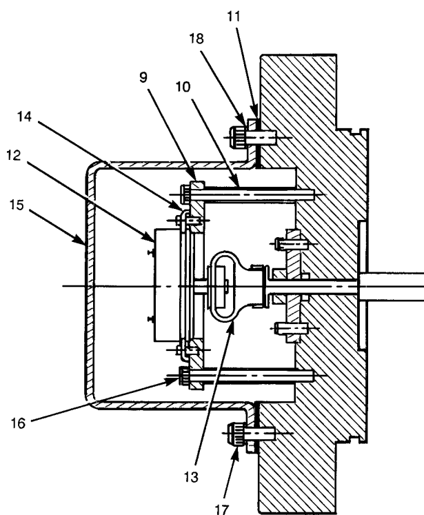
FIG. 3 – VOLUMINIZER POTENTIOMETER PARTS
