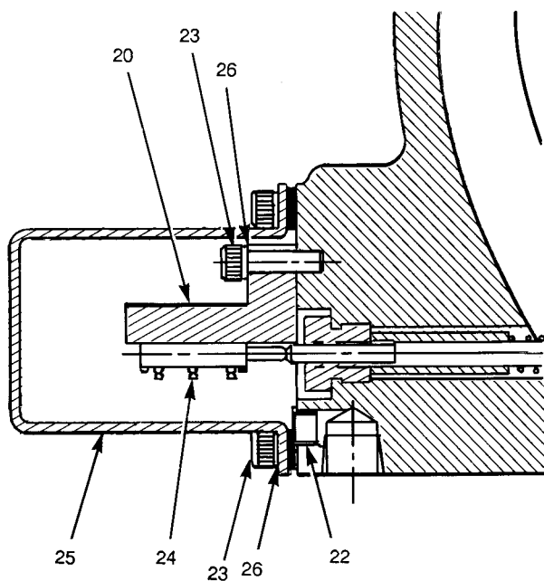
FIG. 3 – VOLUMINIZER POTENTIOMETER PARTS
