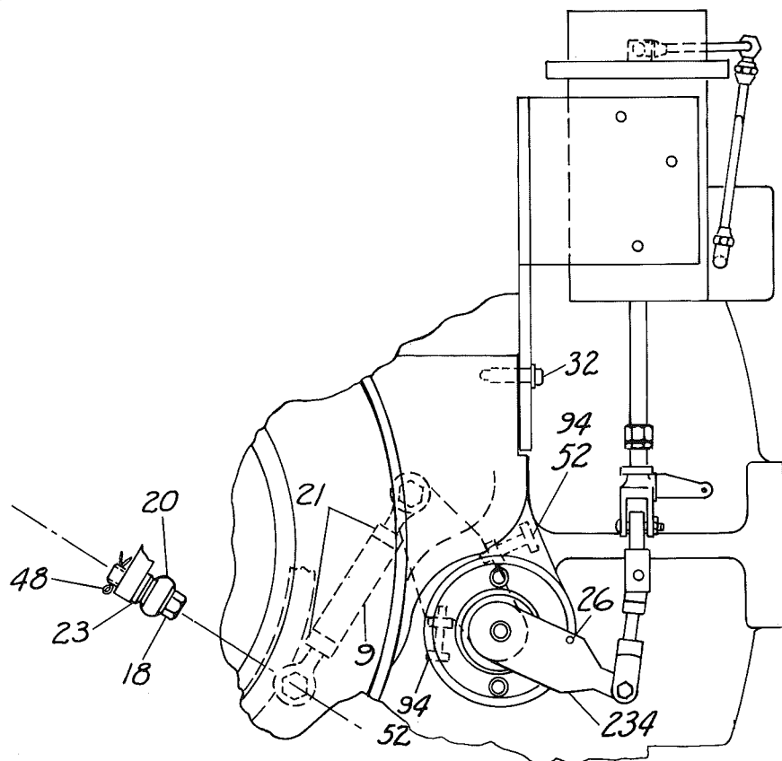
FIG. 7- Air Motor
