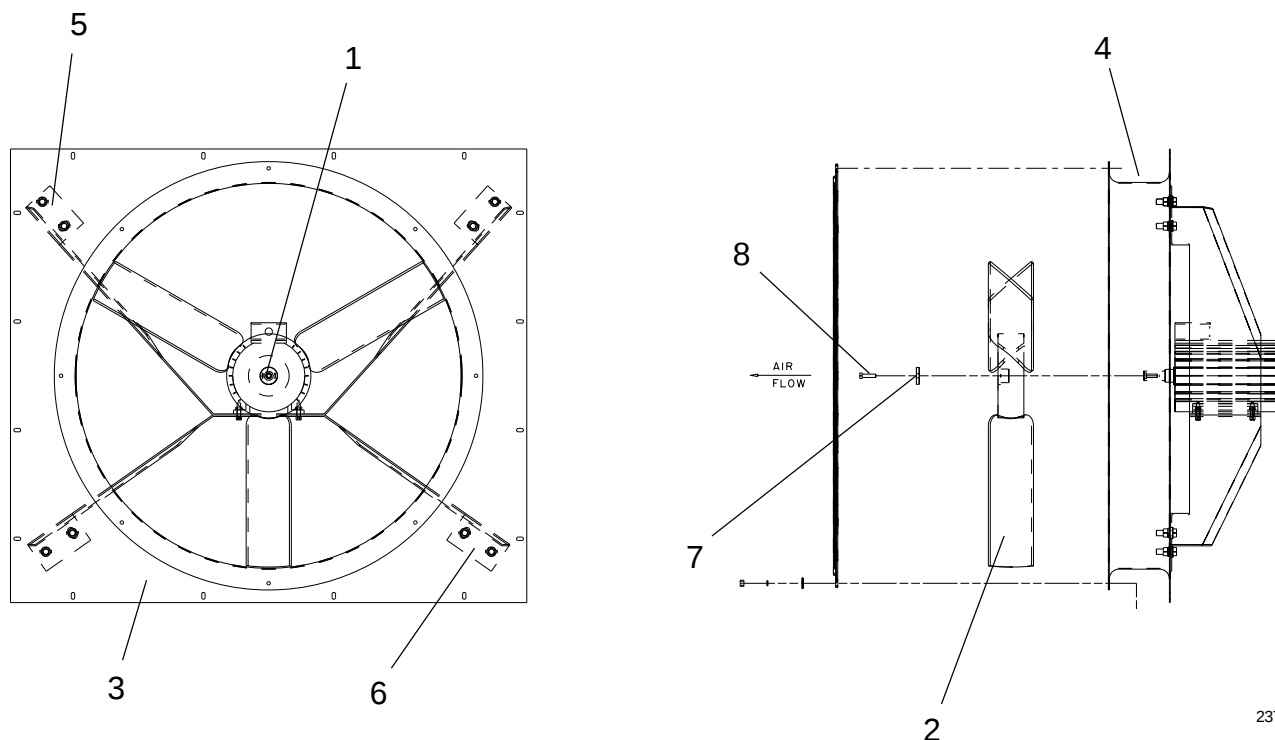
FIG. 4 – FAN COMPONENTS
