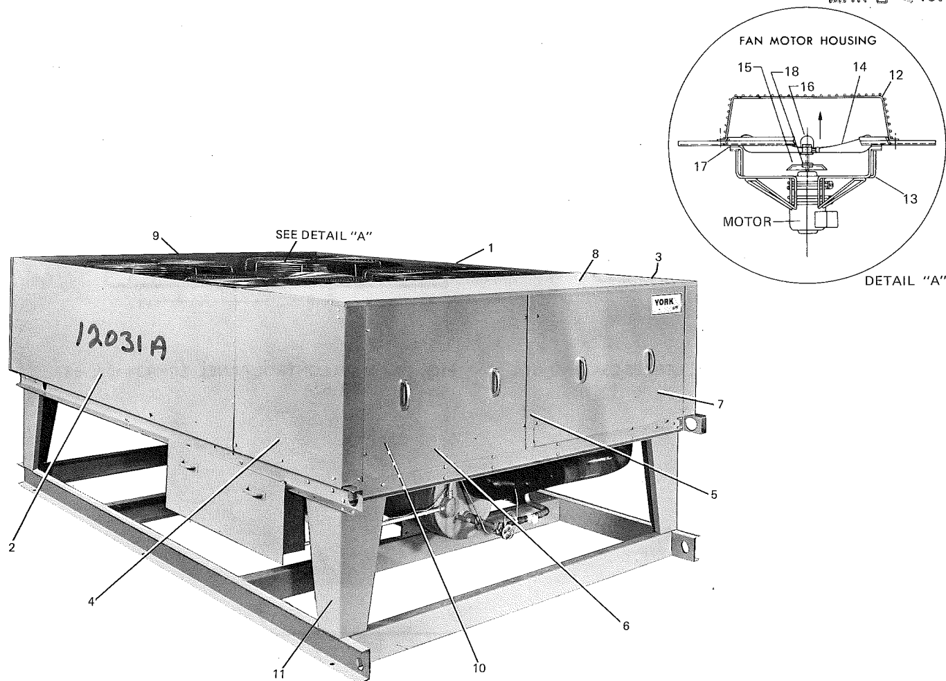
FIG. 1— MODEL LCHA35
