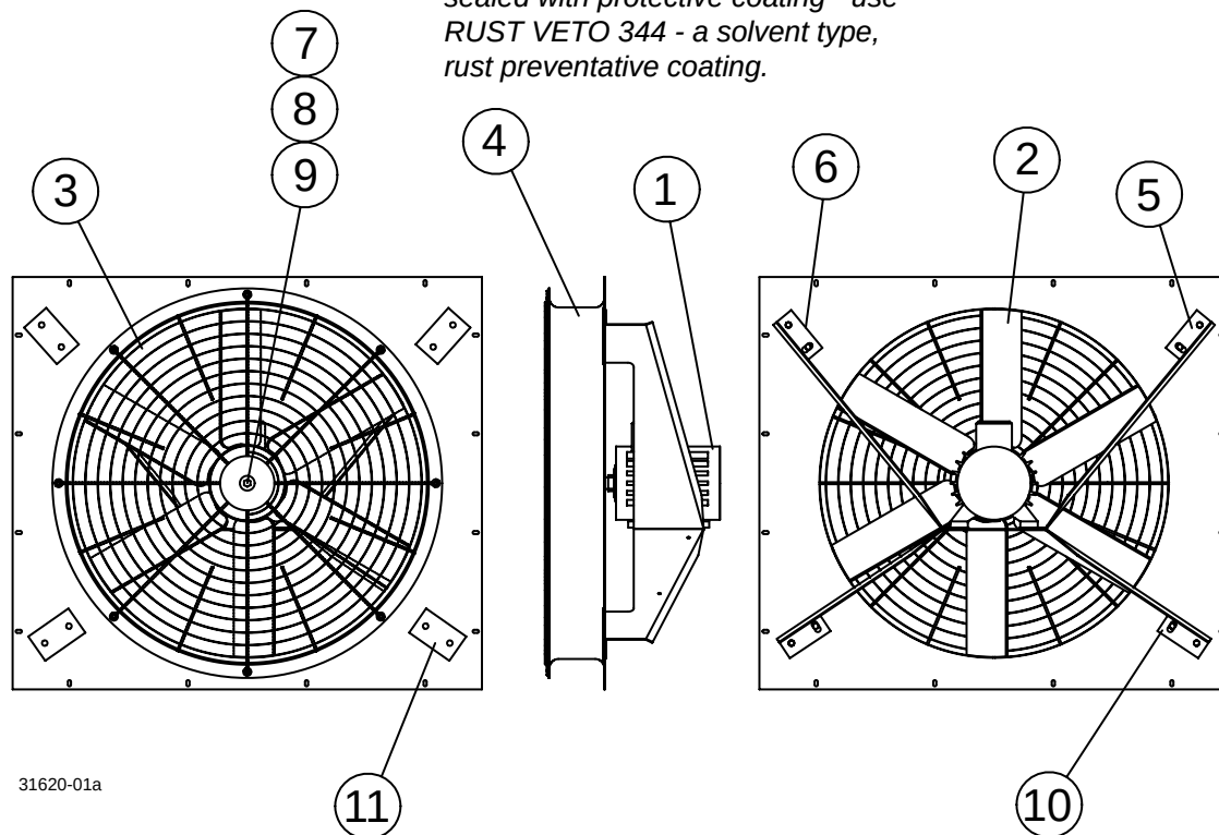
FIG. 3 – FAN COMPONENTS
