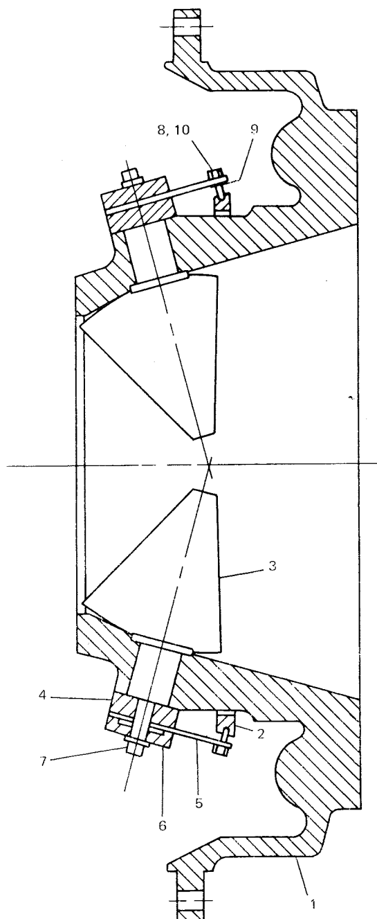
FIG. 7— PRV ASSEMBLY
