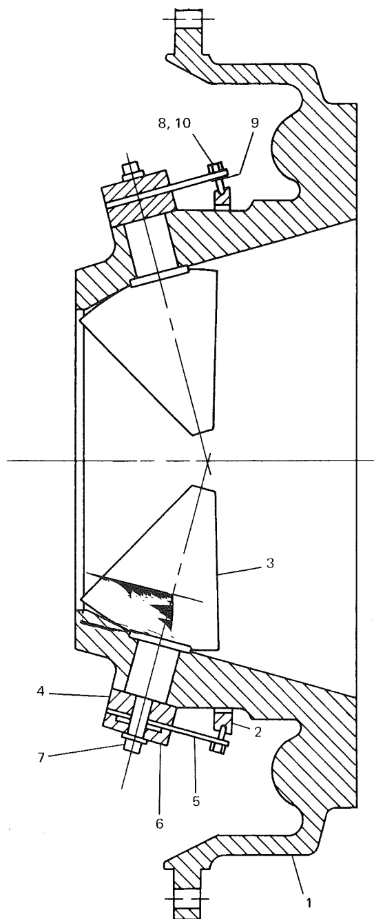
FIG. 7 — PRV ASSEMBLY
