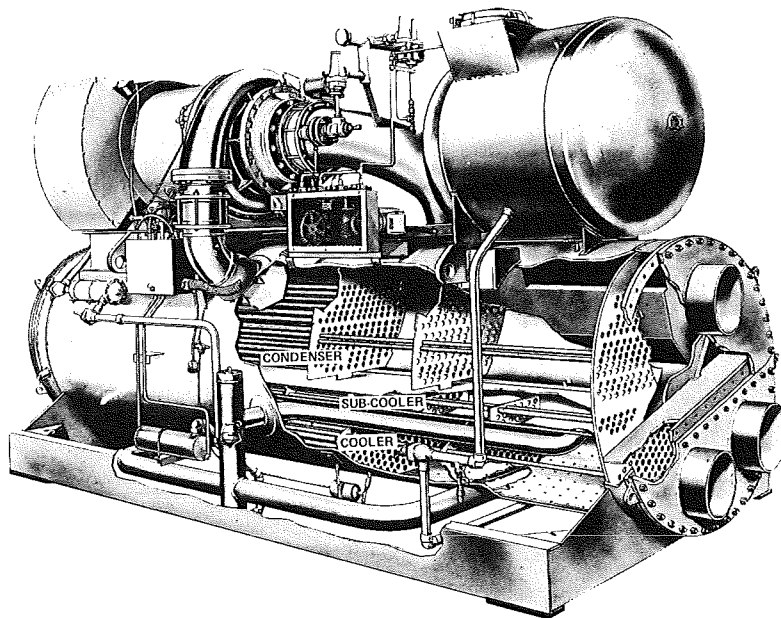
HT TURBOPAK
