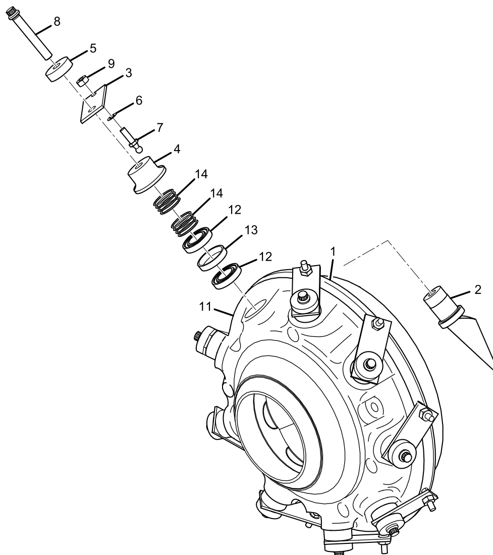
FIG. 17 – COMPRESSOR PRV (K3)
