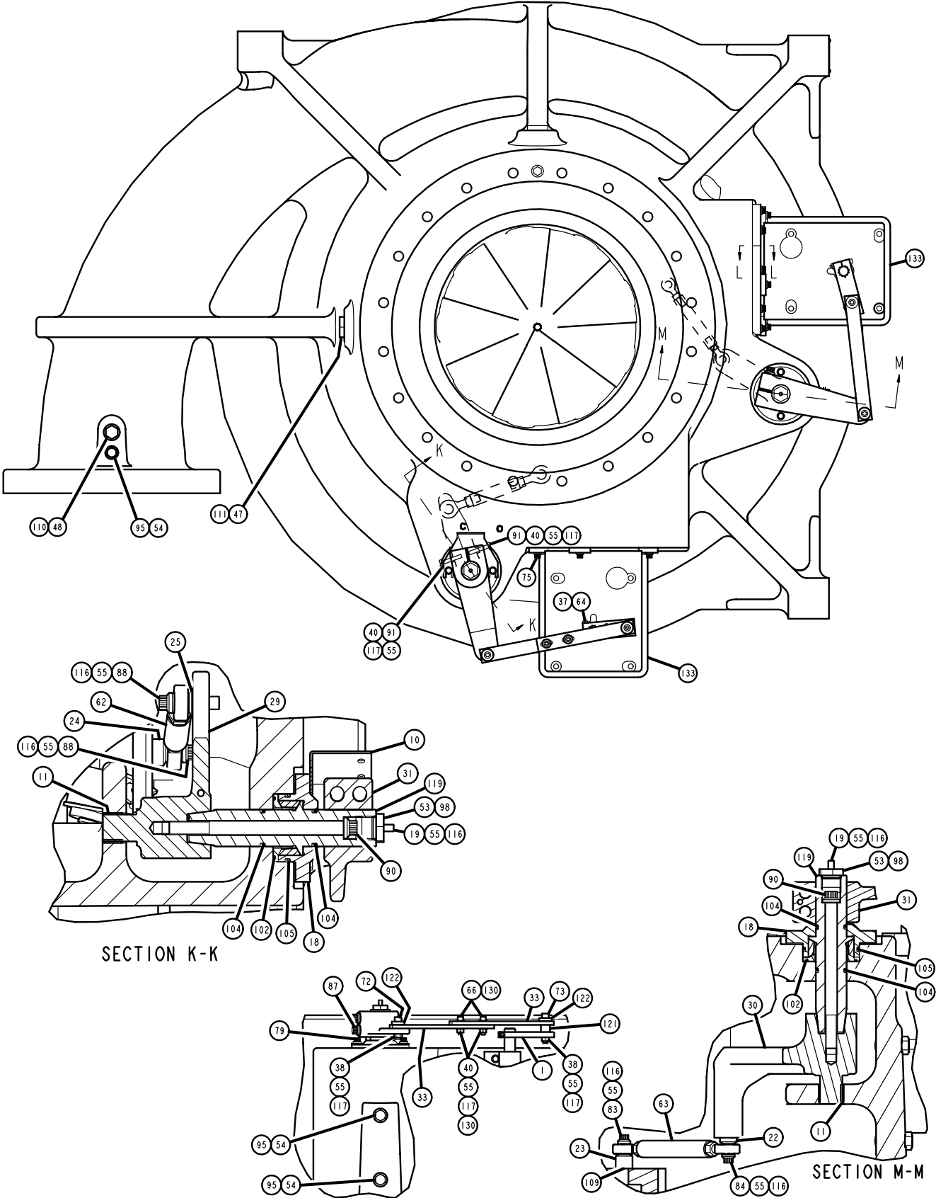
FIG. 15 – K3 COMPRESSOR
