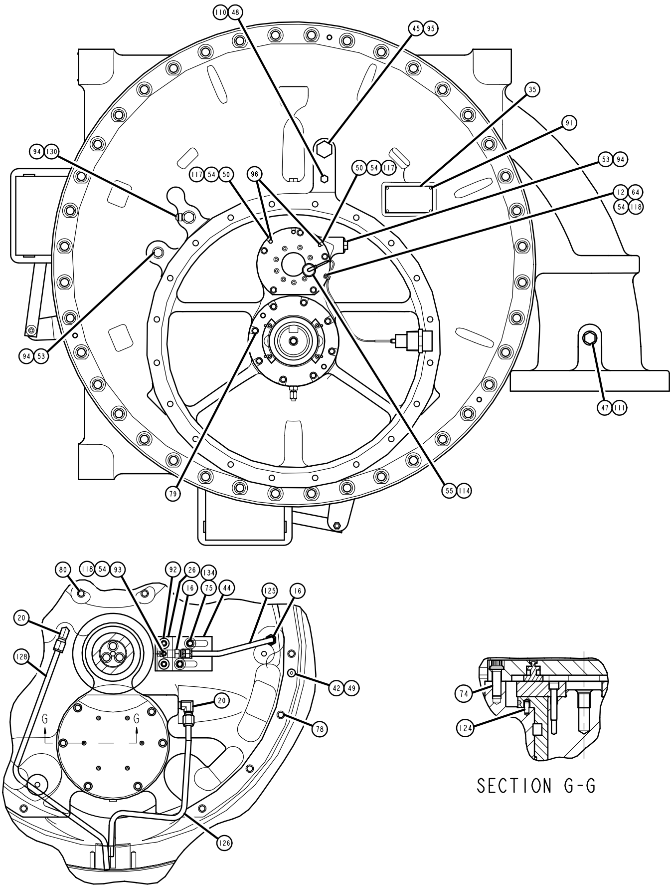
FIG. 2 – K1 COMPRESSOR
