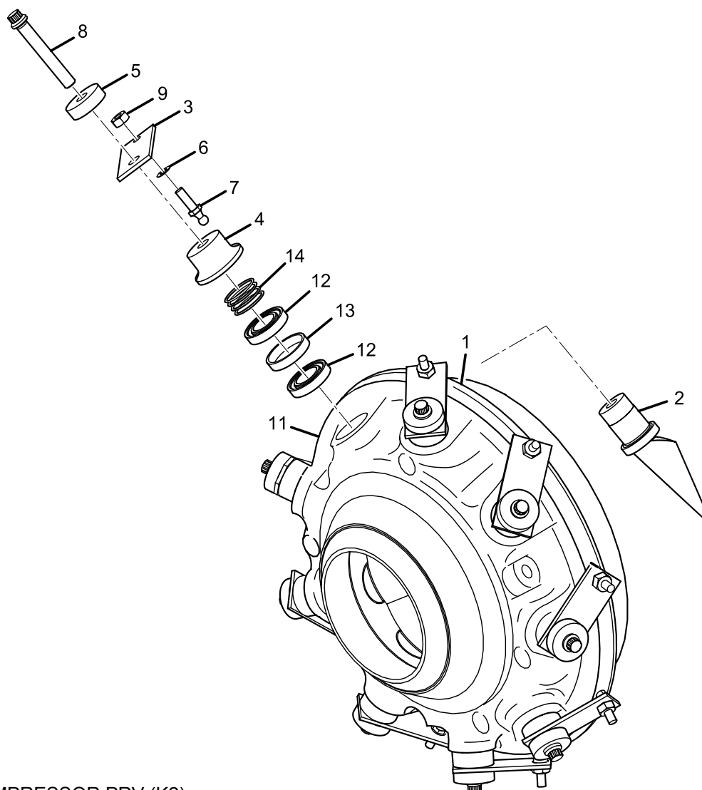
FIG. 11 – COMPRESSOR PRV (K2)
