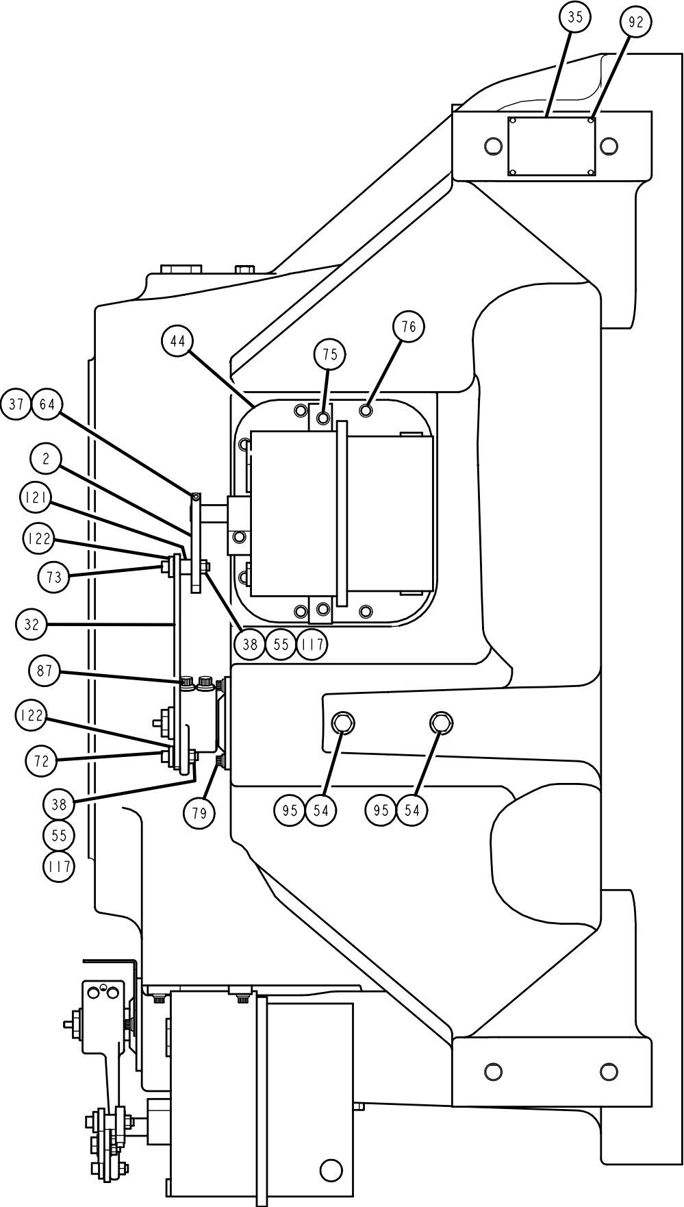
FIG. 16 – K3 COMPRESSOR
