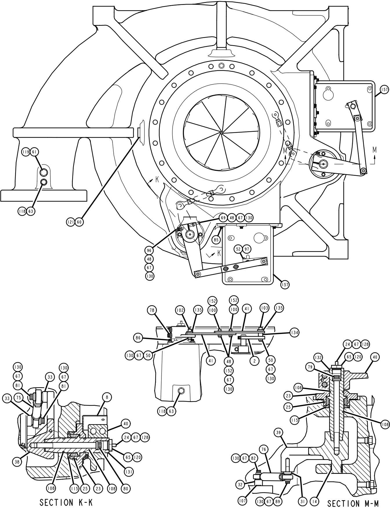
FIG. 9 – K2 COMPRESSOR
