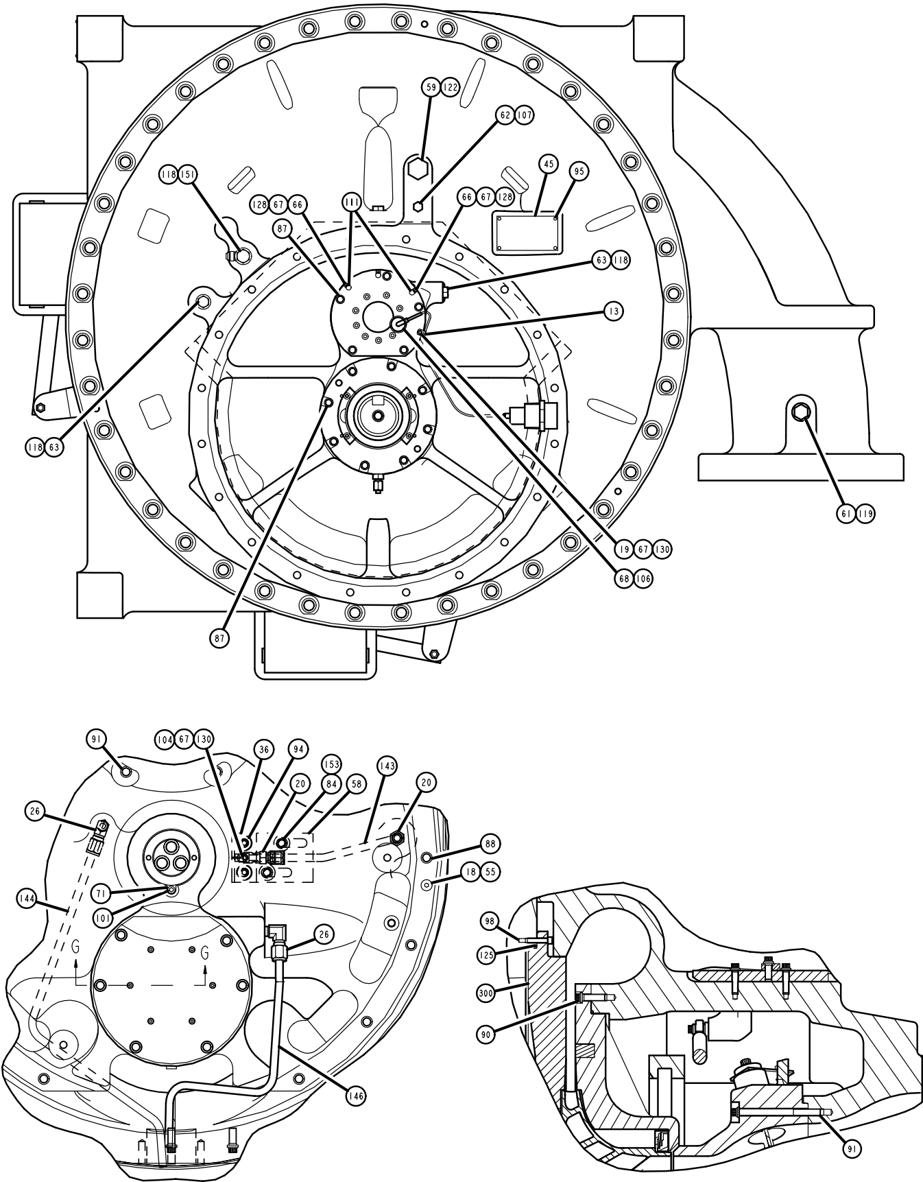
FIG. 8 – K2 COMPRESSOR
