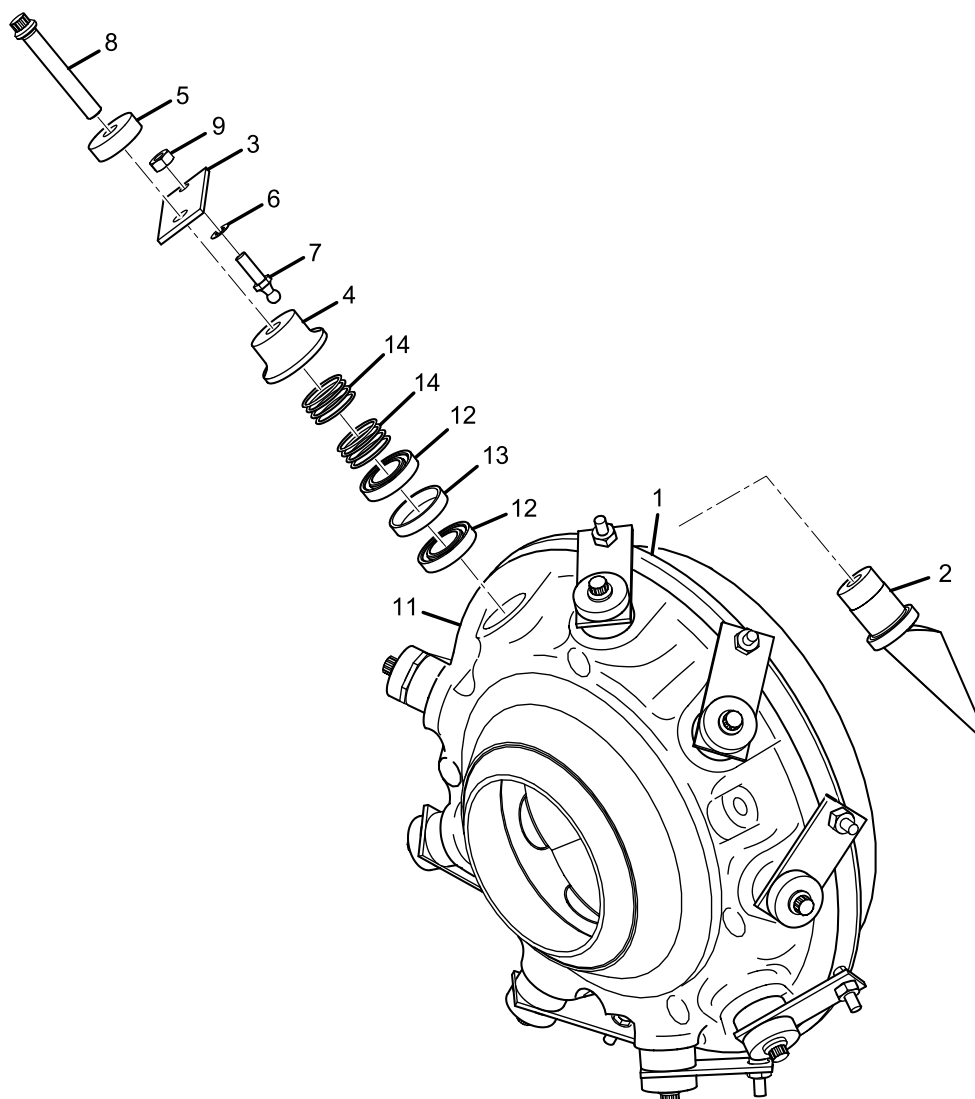
FIG. 23 – COMPRESSOR PRV (K4)
