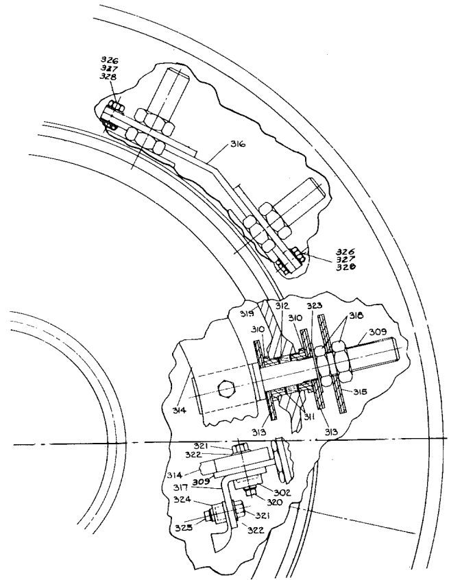
FIG. 6— Motor Terminals
