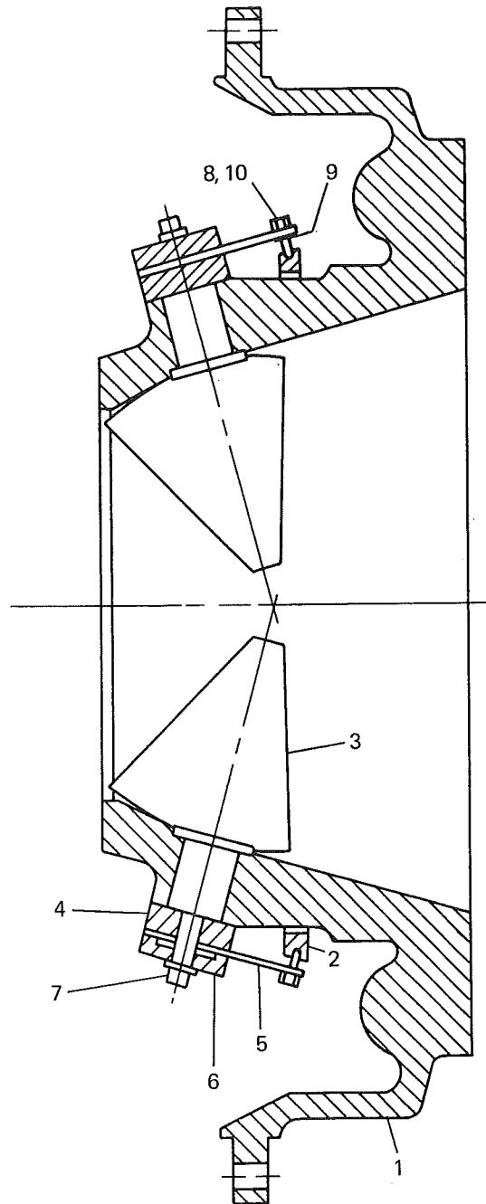
FIG. 7— PRV ASSEMBLY
