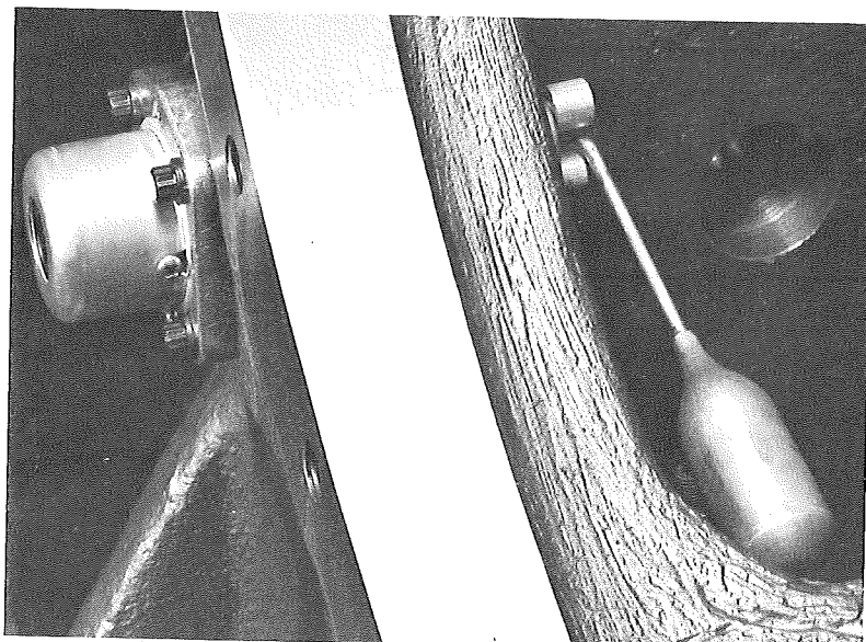
FIG. 14— FLOAT SWITCH
