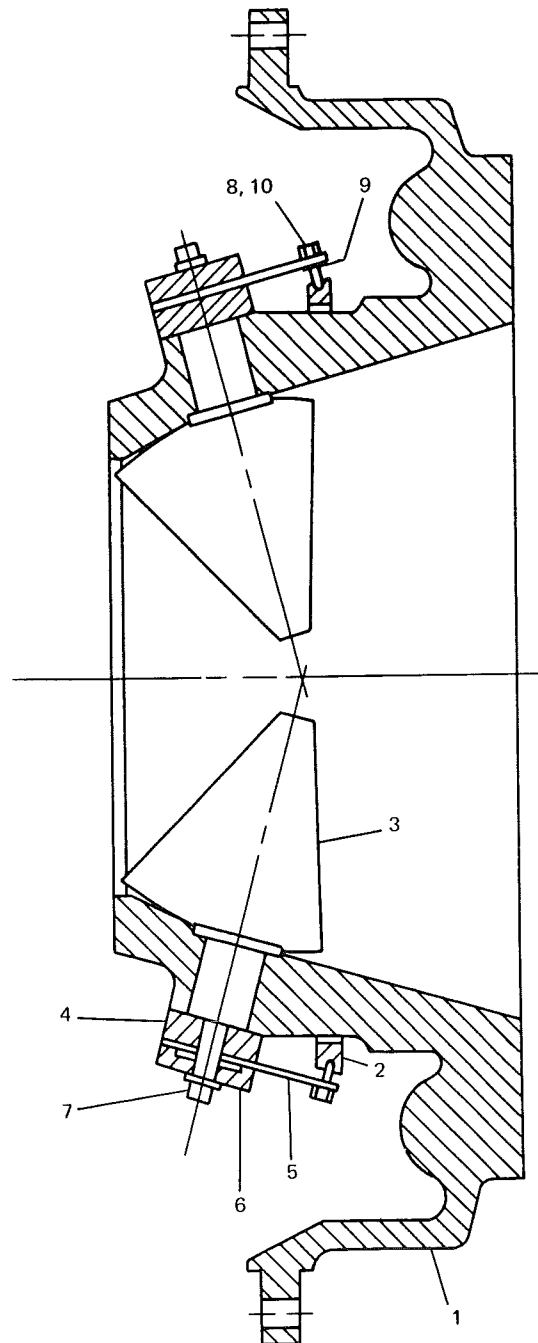
FIG. 7— PRV ASSEMBLY
